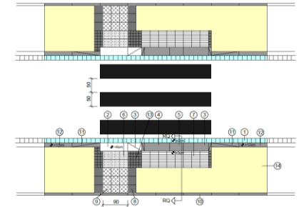
Ansicht Bordsteine M 1:50
