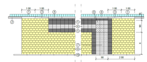
Systemplan Bushaltestelle, M 1:50
